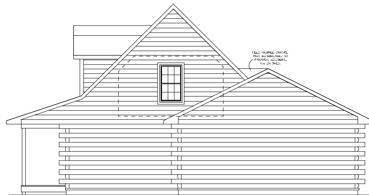
RIGHT ELEVATION SCALE: 1/8" = 1'-0"
